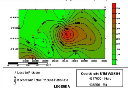
Tendința de evoluție a concentrației "total produse petroliere" (adâncimea de prelevare - 15 cm, concentrații în mg/kg sol uscat "total produse petroliere").
